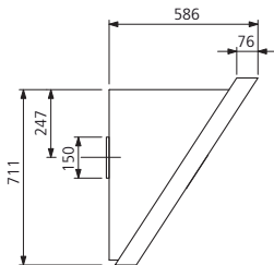
Seitenansicht
